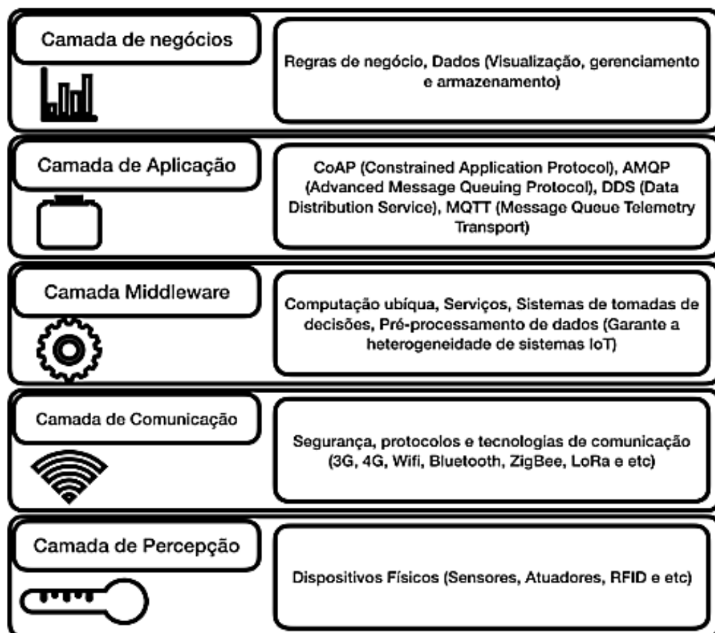
Figura 3 - Arquitetura de uma solução IoT.
