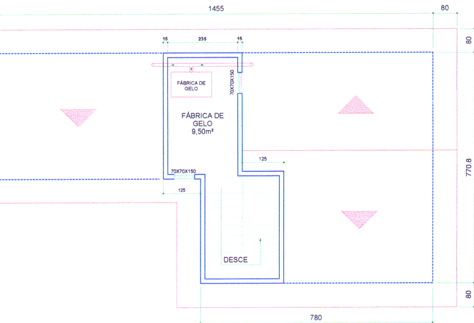
PLANTA BAIXA PVTO SUPERIOR S/ ESC – A: 19,50m 2
